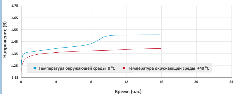
Заряд током C/5 при различных температурах
