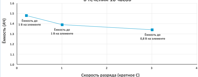
Допустимая разрядная ёмкость после заряда током C/10 в течении 16 часов
