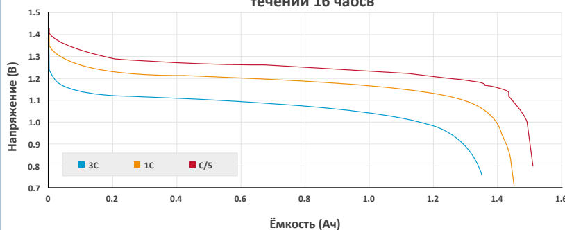
Допустимая разрядная ёмкость после заряда током C/10 в течении 16 часов
