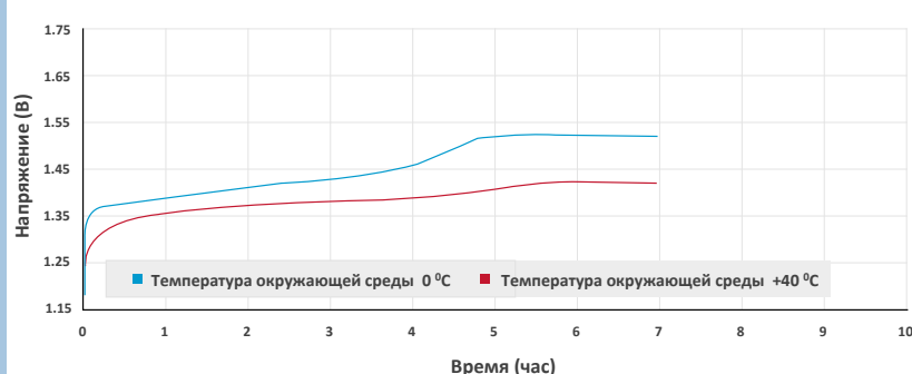
Разрядная ёмкость различными токами после заряда током C/10 в течении 16 часов
