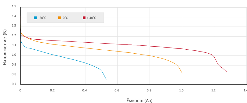
Разрядная ёмкость током 1.5 А при разных температурах, после заряда током 1С
