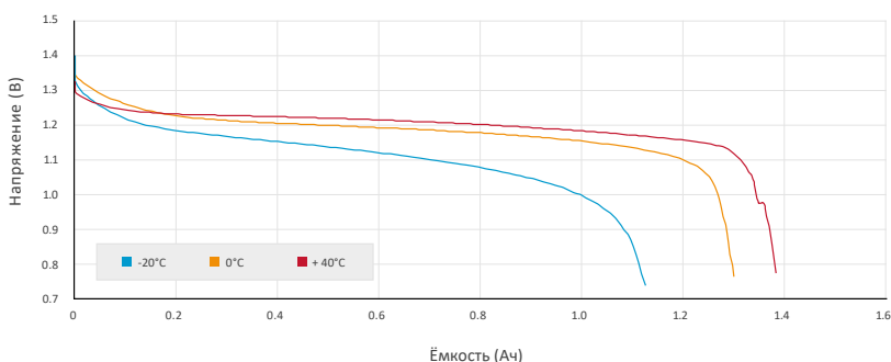
Разрядная ёмкость током 1.5 А при разных температурах, после заряда током 1С
